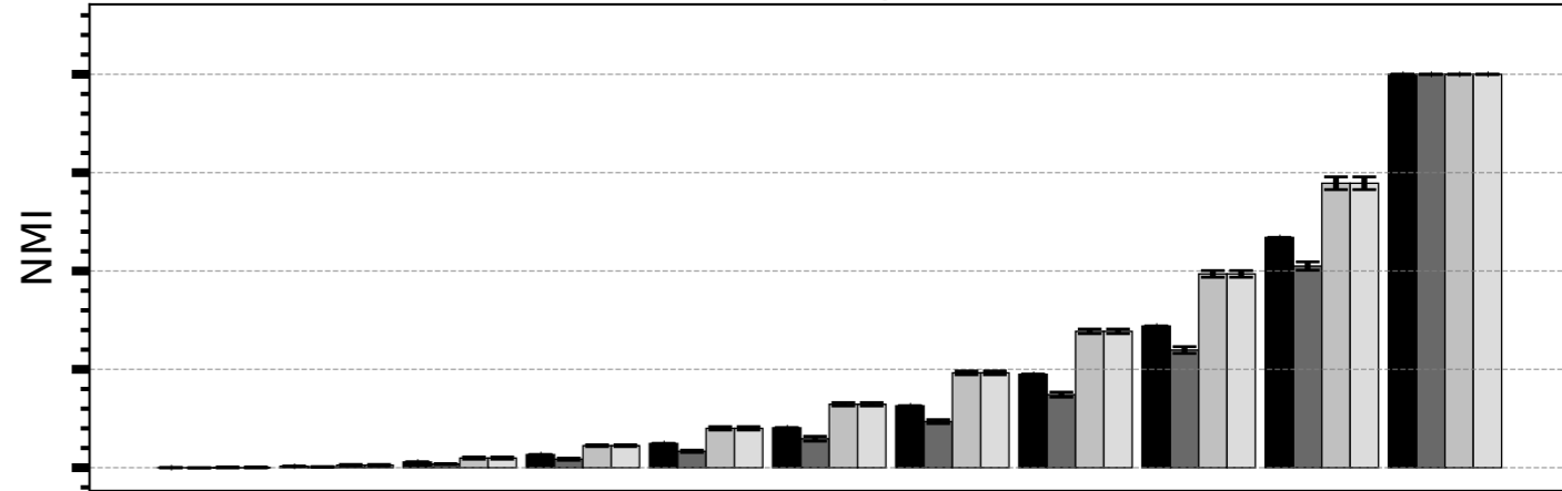
Dimensionality (d) = 4
