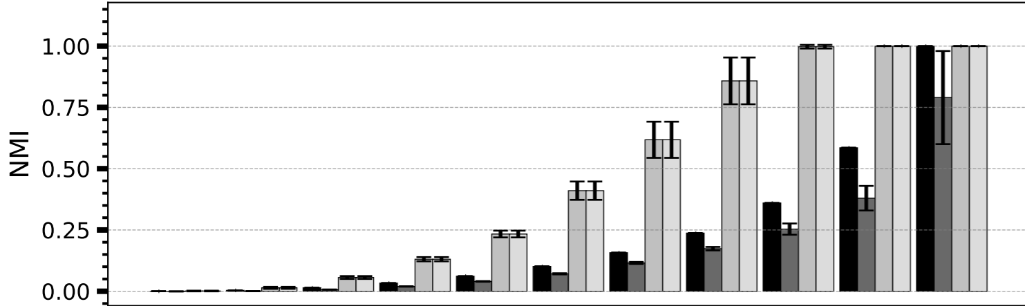
Dimensionality (d) = 16
