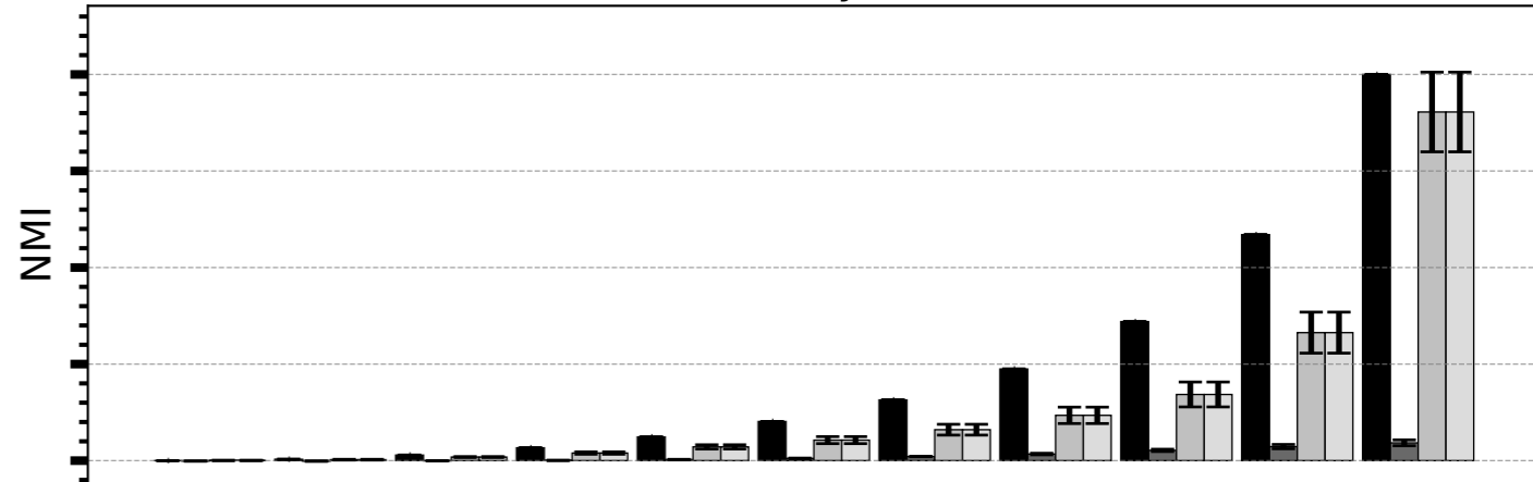
Dimensionality (d) = 128
