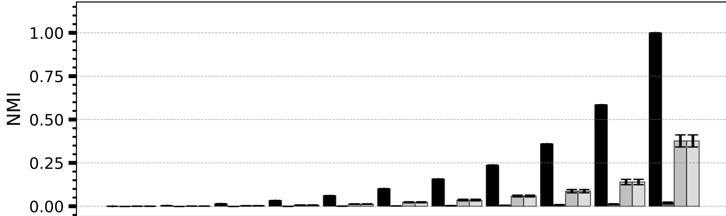
Dimensionality (d) = 256
